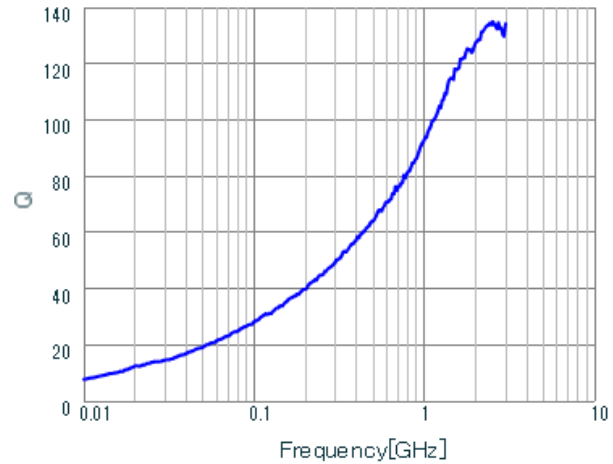
LQW18AN4N3B8Z Q.
