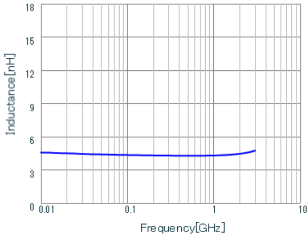
LQW18AN4N3B8Z L.
