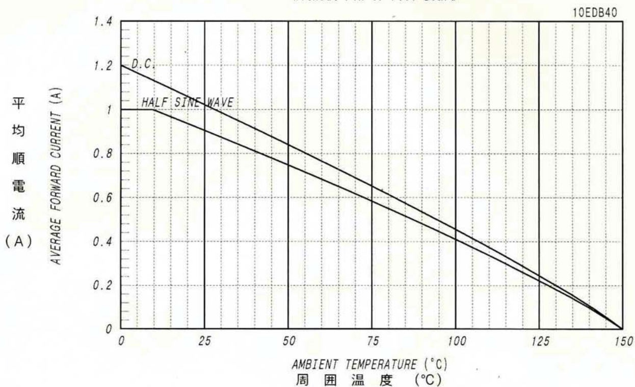
平均順電流 - 周圍溫度定格 AVERAGE FORWARD CURRENT VS. AMBIENT TEMPERATURE
