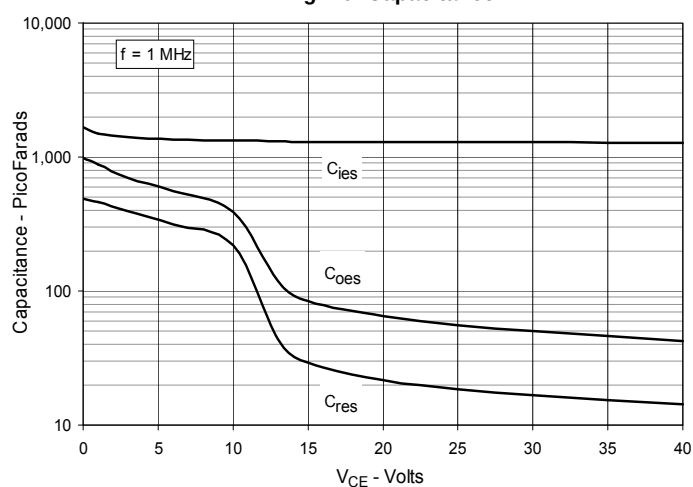
Fig. 10. Capacitance
