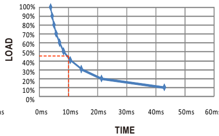
DDR-120B-24
