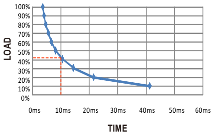
DDR-120B-12
