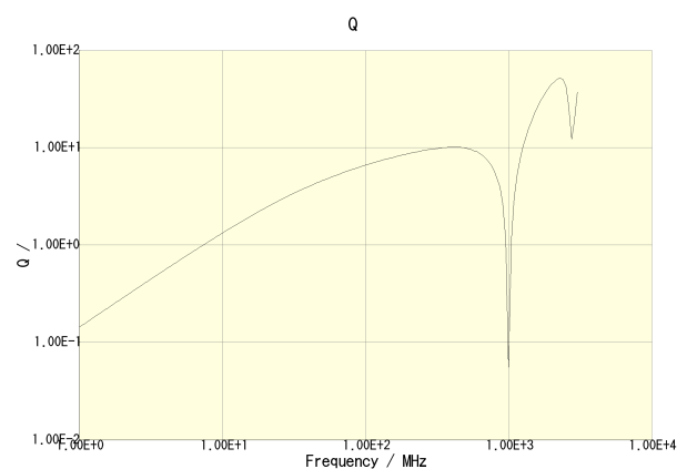
MLG0603SR11JT000
