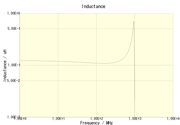
MLG0603SR11JT000
