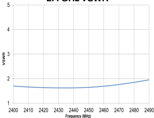
2.4 GHz VSWR
