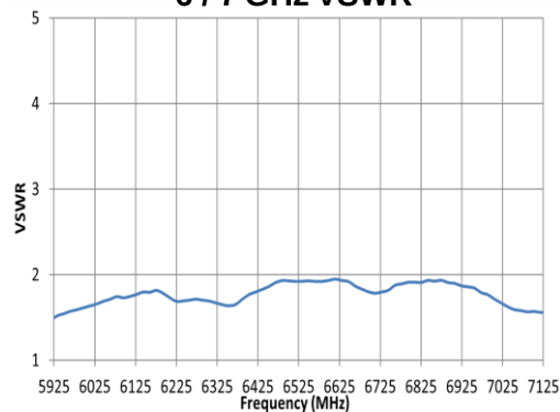
6 / 7 GHz VSWR
