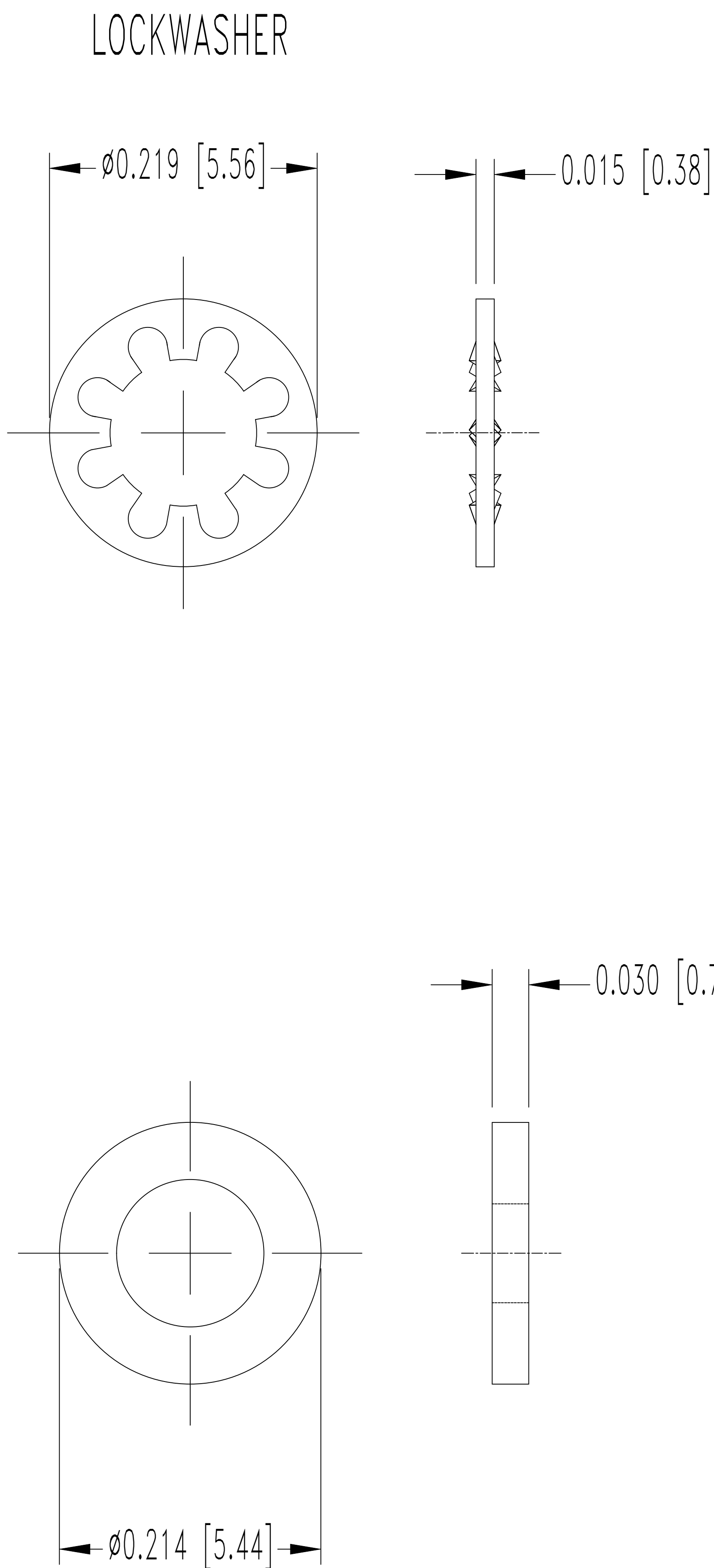
LOCKWASHER
