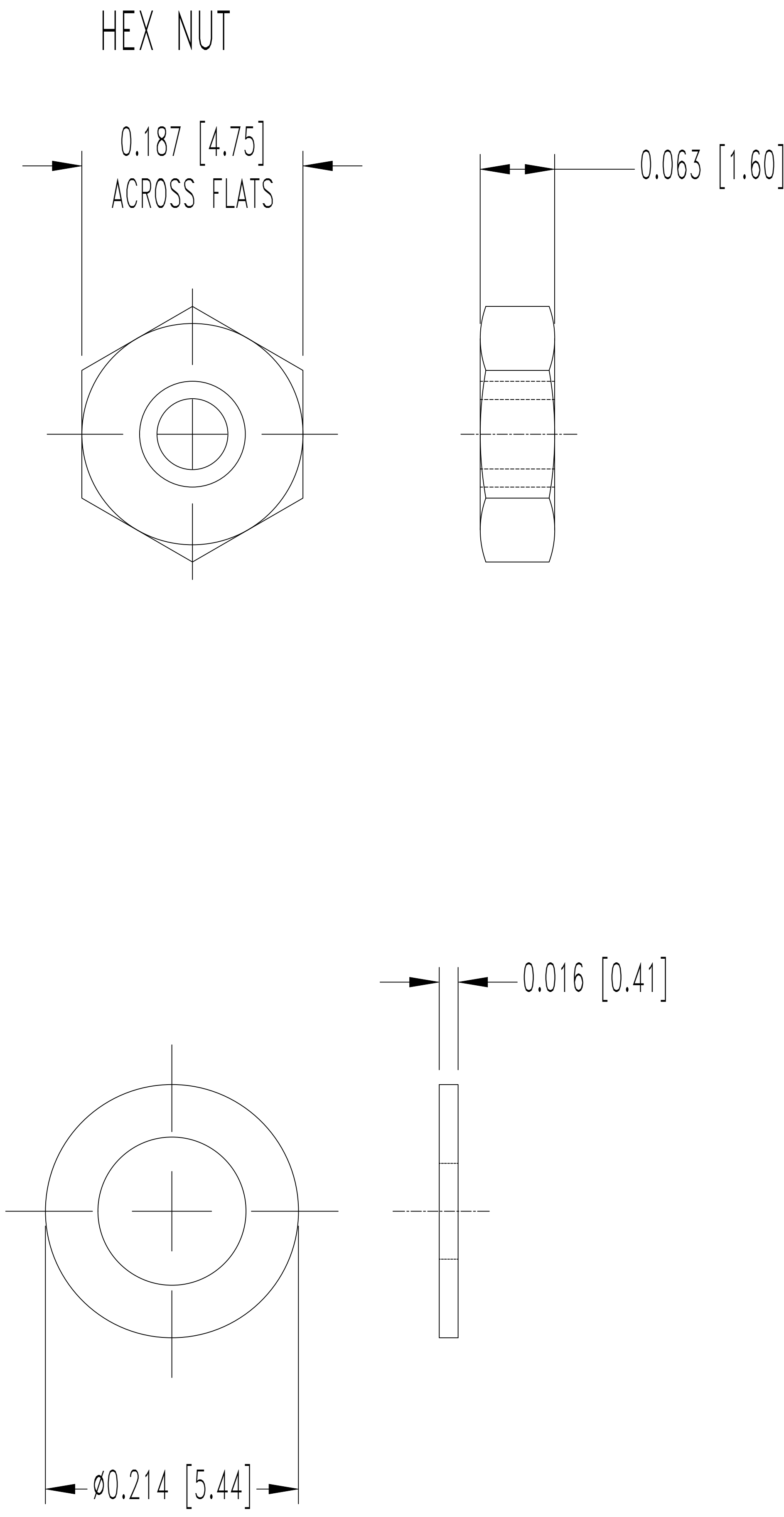
HEX NUT
