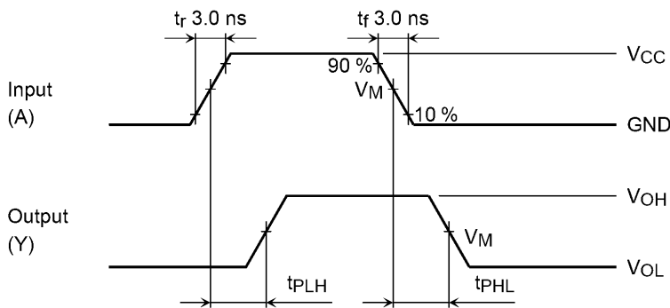
Fig. 9.8.1 t_{PLH} , t_{PHL}
