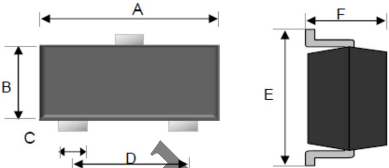
SOT-323
