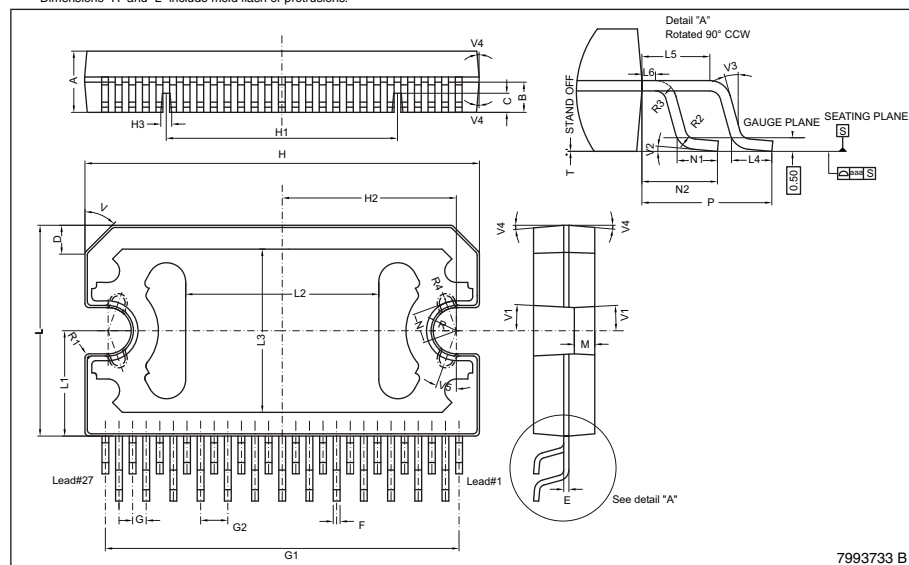
DIM. mm inch MIN. TYP. MAX. MIN. TYP. MAX. A 4.45 4.50 4.65 0.1752 0.1772 0.1831 B 2.12 2.22 2.32 0.0835 0.0874 0.0913 C 1.40 0.0551 D 2.00 0.0787 E 0.36 0.40 0.44 0.0142 0.0157 0.0173 F(**) 0.47 0.51 0.57 0.0185 0.0201 0.0224 G(*) 0.75 1.00 1.25 0.0295 0.0394 0.0492 G1 25.70 26.00 26.30 1.0118 1.0236 1.0354 G2(*) 1.75 2.00 2.25 0.0689 0.0787 0.0886 H(**) 28.85 29.23 29.40 1.1358 1.1508 1.1575 H1 17.00 0.6693 H2 12.80 0.5039 H3 0.80 0.0315 L(**) 15.50 15.70 15.90 0.6102 0.6181 0.6260 L1 7.70 7.85 7.95 0.3031 0.3091 0.3130 L2 14.00 14.20 14.40 0.5512 0.5591 0.5669 L3 11.80 12.00 12.20 0.4646 0.4724 0.4803 L4 1.30 1.48 1.66 0.0512 0.0583 0.0654 L5 2.42 2.50 2.58 0.0953 0.0984 0.1016 L6 0.42 0.50 0.58 0.0165 0.0197 0.0228 M 1.50 0.0591 N 2.20 0.0866 N1 1.30 1.48 1.66 0.0512 0.0583 0.0654 N2(*) 2.73 2.83 2.93 0.1075 0.1114 0.1154 P(*) 4.73 4.83 4.93 0.1862 0.1902 0.1941 R 1.70 0.0669 R1 0.30 0.0118 R2 0.35 0.40 0.45 0.0138 0.0157 0.0177 R3 0.35 0.40 0.45 0.0138 0.0157 0.0177 R4 0.50 0.0197 T(*) -0.08 0.10 -0.0031 0.0039 aaa(*) 0.1 0.0039 V 45° 45° V1 3° 3° V2 3° 5° 7° 3° 5° 7° V3 12° 15° 18° 12° 15° 18° V4 5° 5° V5 20° 20°
