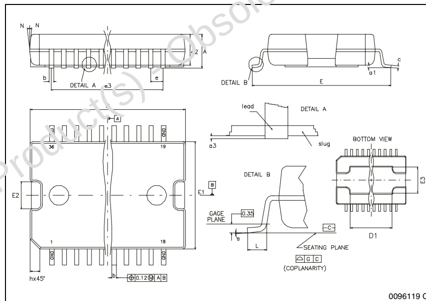
PowerSO-36
