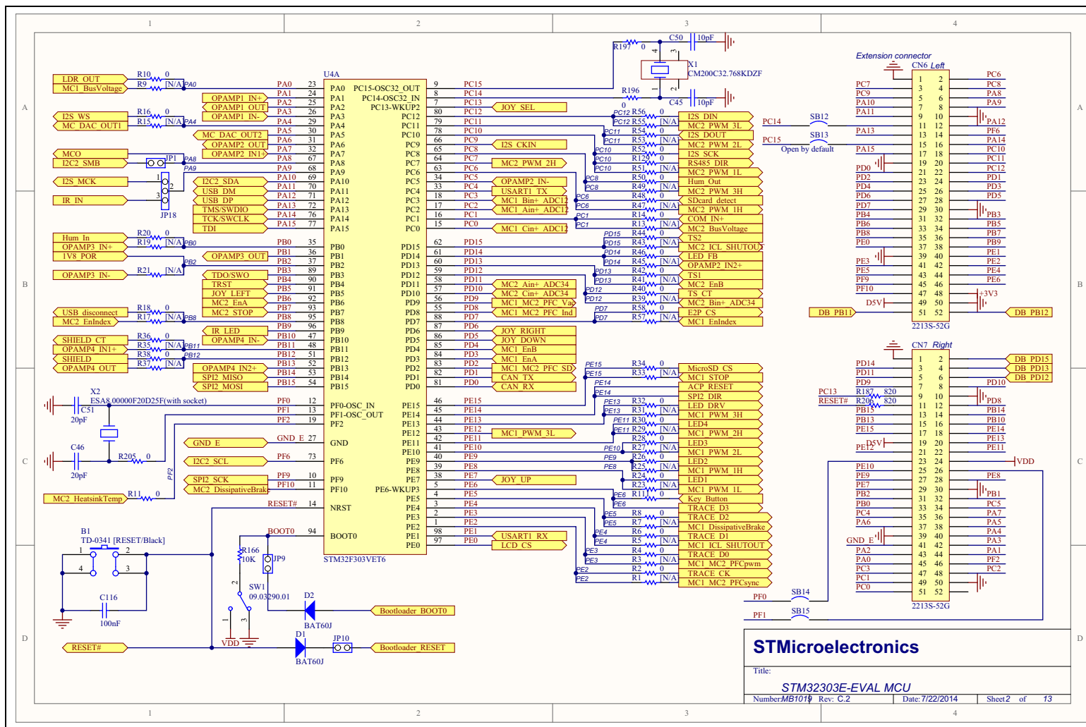
Figure 19. STM32303E-EVAL MCU
