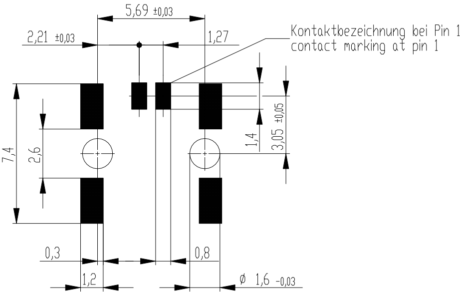
Leiterplatten-Layout für SMT PCB-Layout for SMT
