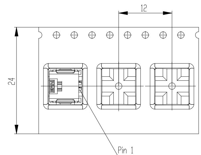
Abspulrichtung - reel off direction
