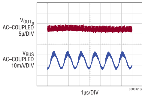
V_{\text{OUTn}} Noise Waveform V_{\text{OUTn}} : 10Hz to 100kHz BW V_{\text{BUS}} : Wideband
