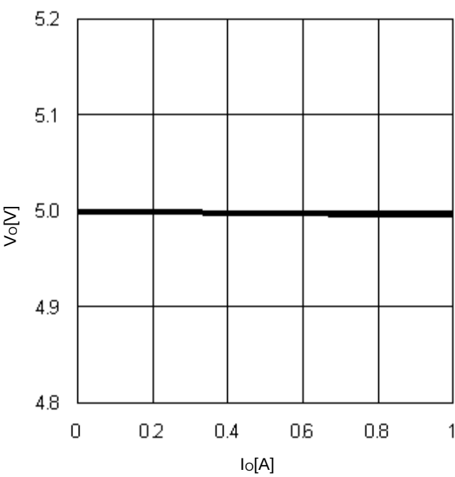
Fig.13 I_o - V_o
