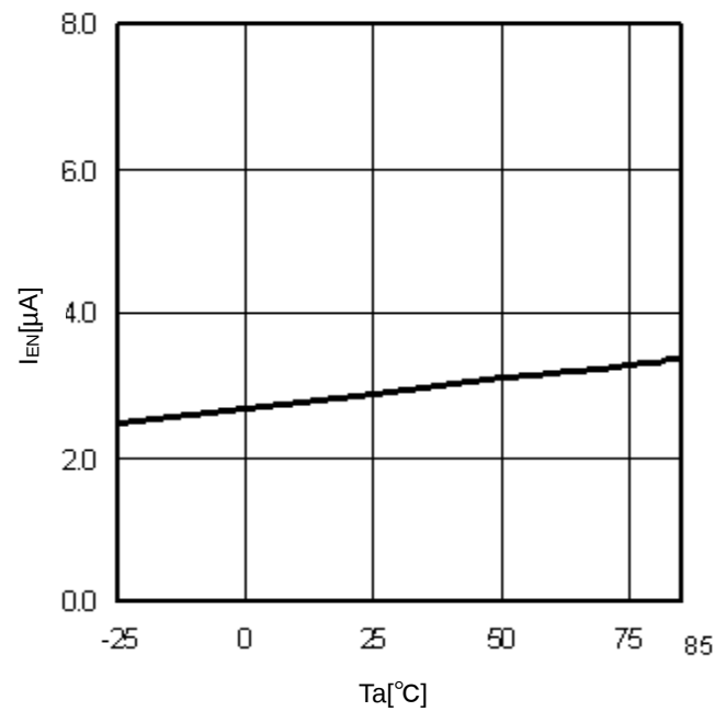
Fig.12 T_a - I_{EN}
