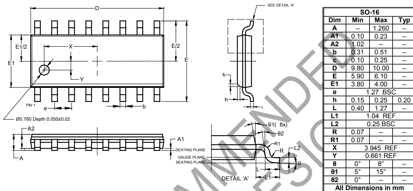
SO-16
