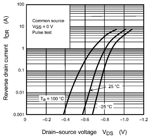
Fig. 8.9 I_{DR} - V_{DS}
