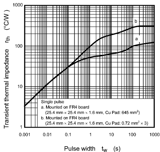
Fig. 8.13 r_{th} - t_w
