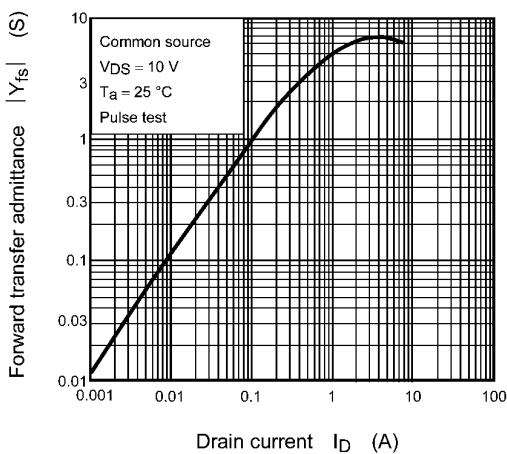
Fig. 8.8 |Y_{fs}| - I_D
