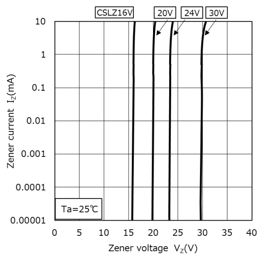
I_Z - V_Z (2)
