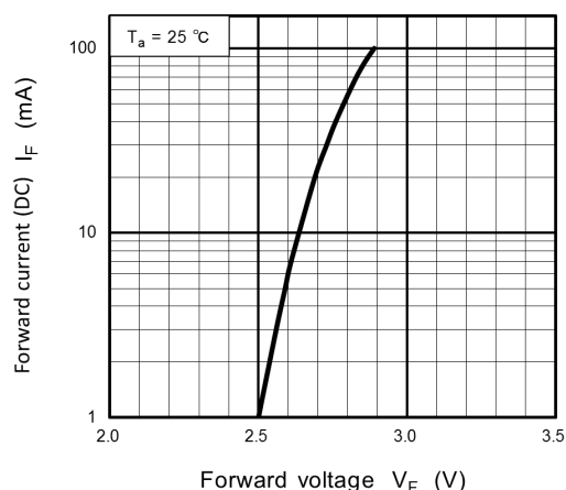
Fig. 8.1 I_F - V_F
