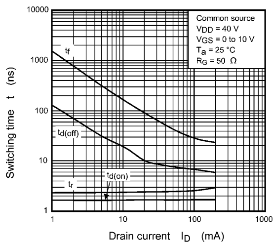
Fig. 8.10 t - I_D
