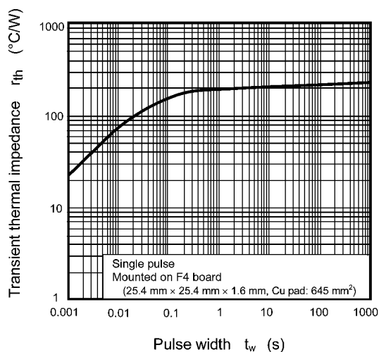
Fig. 8.11 r_{th} - t_w
