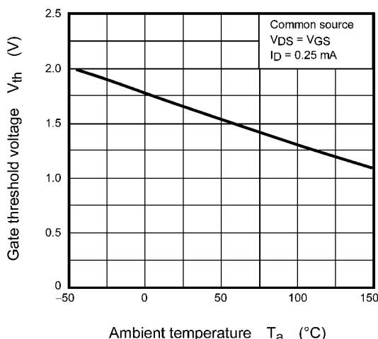
Fig. 8.6 V_{th} - T_a
