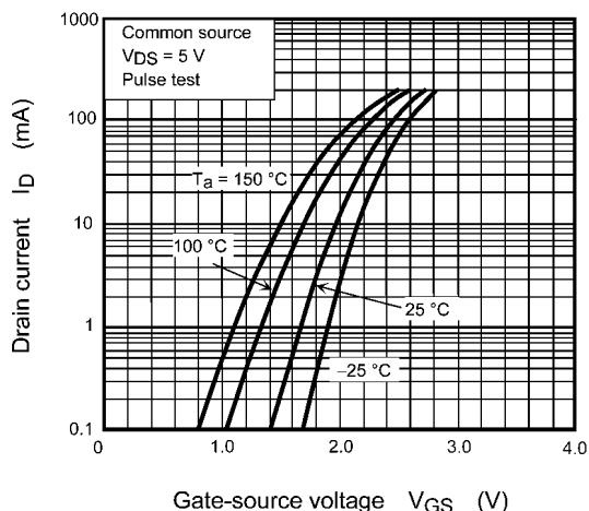
Fig. 8.2 I_D - V_{GS}
