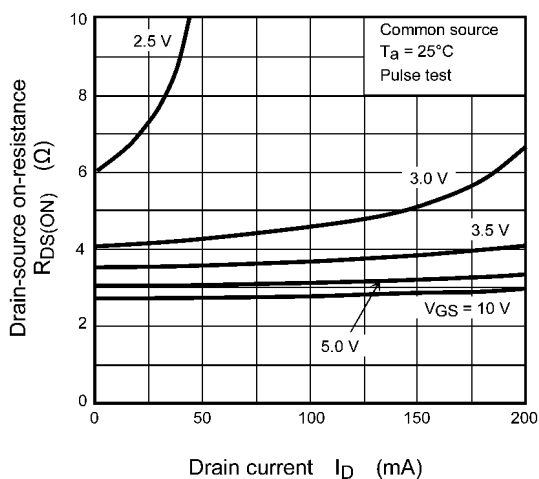
Fig. 8.3 R_{DS(ON)} - I_D
