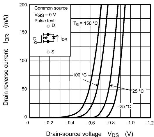
Fig. 8.8 I_{DR} - V_{DS}
