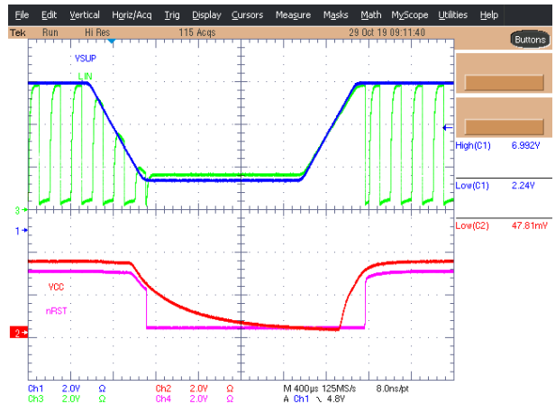
Figure 10-9. TLIN1028S-Q1 Brownout
