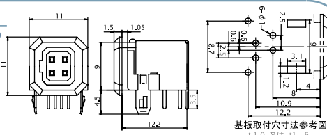
基板取付穴寸法参考図 (t1.0又はt1.6)
