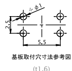
基板取付穴寸法参考図 (t1.6)
