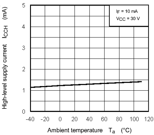
Fig. 12.2.6 I_{cCH} - T_a
