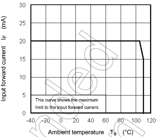
Fig. 12.2.2 I_F - T_a
