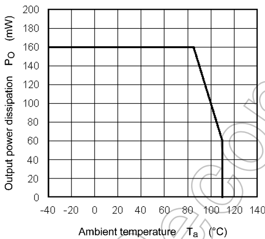
Fig. 12.2.3 P_O - T_a
