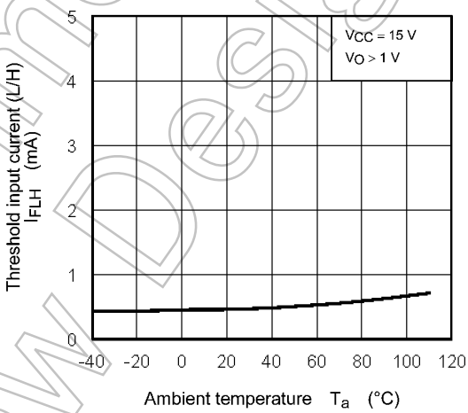
Fig. 12.2.4 I_{FLH} - T_a
