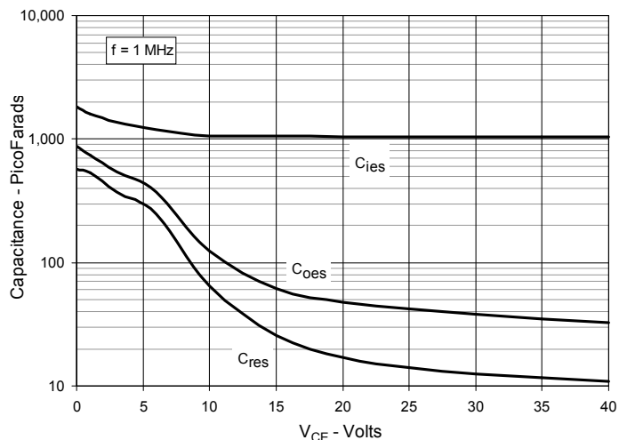
Fig. 10. Capacitance
