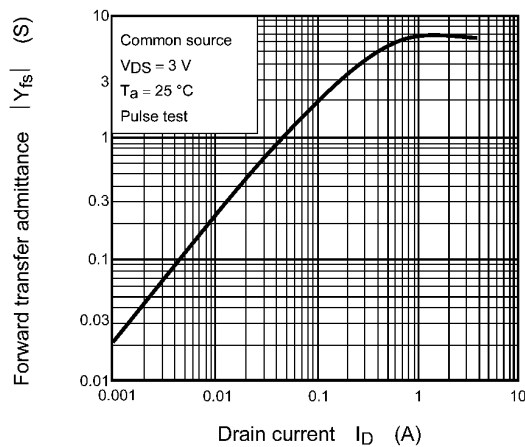
Fig. 7.1.8 |Y_{fs}| - I_D
