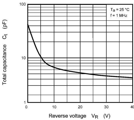
Fig. 7.2.3 C_t - V_R
