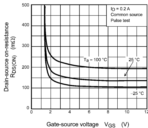
Fig. 7.1.3 R_{DS(ON)} - V_{GS}
