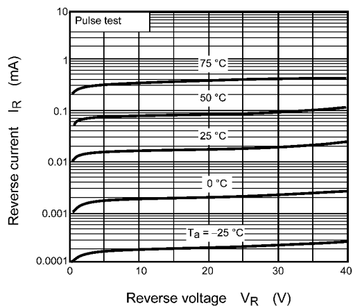
Fig. 7.2.2 I_R - V_R
