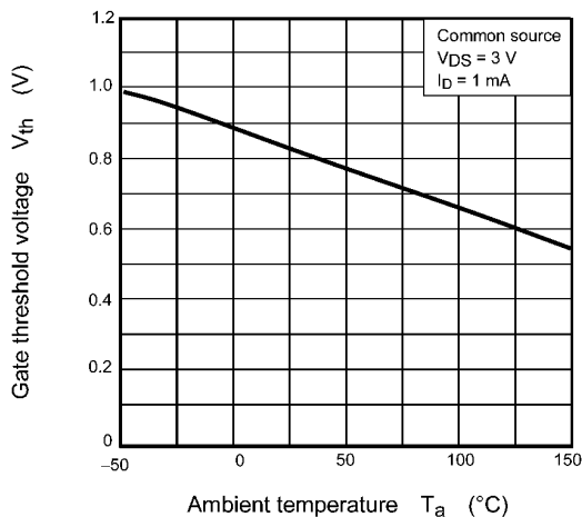
Fig. 7.1.7 V_{th} - T_a
