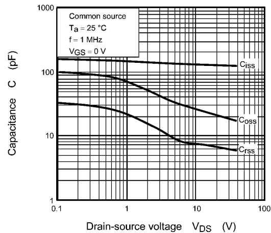
Fig. 7.1.10 C - V_{DS}
