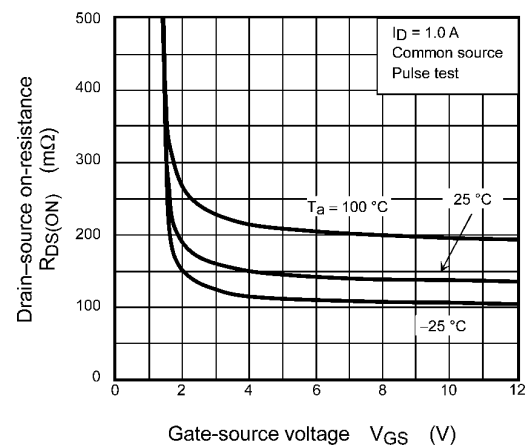
Fig. 7.1.4 R_{DS(ON)} - V_{GS}
