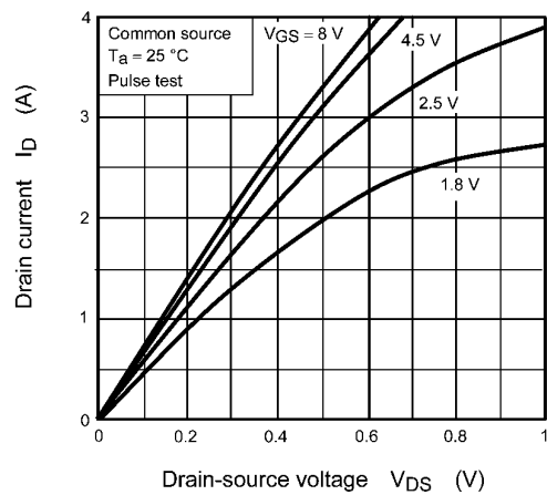
Fig. 7.1.1 I_D - V_{DS}
