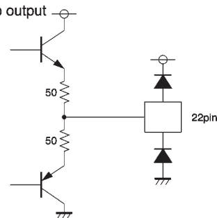
Op-amp output
