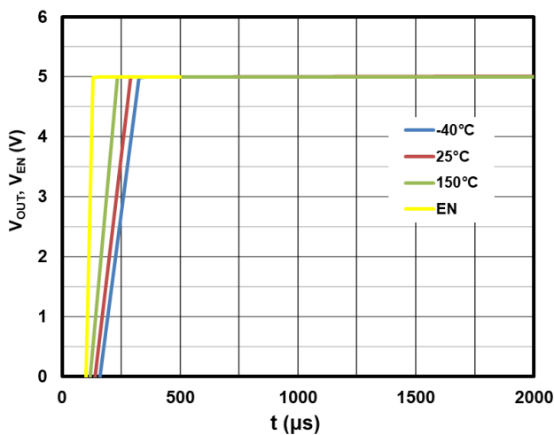
Figure 11. Output Voltage vs. time (EN switched ON)
