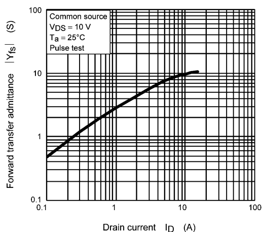
Fig. 8.5 |Y_{fs}| - I_D
