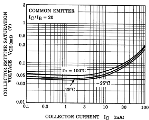
Fig. 9.8 RN1313 V_{CE(sat)}-I_C
