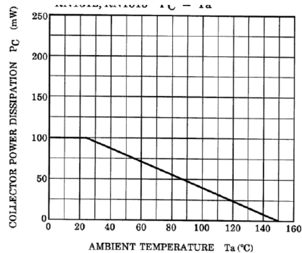
Fig. 9.9 RN1312,RN1313 P_C-T_a
