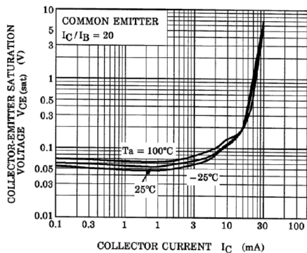
Fig. 9.7 RN1312 V_{CE(sat)}-I_C
