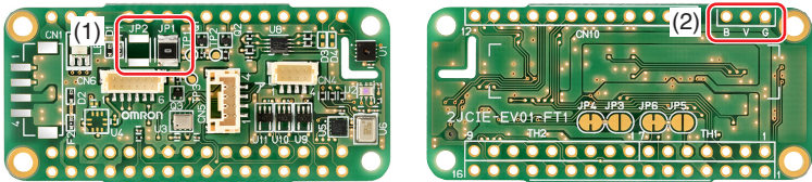
2JCIE-EV01-FT1 Layout
