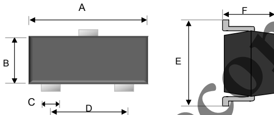
SOT-523
