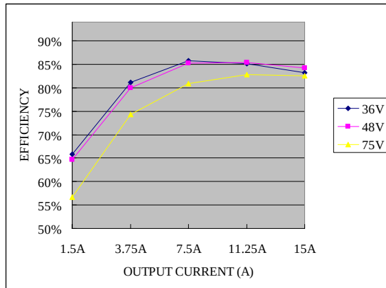
Vo=1.2 V
