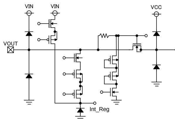
&lt; VOUT Pin &gt;
