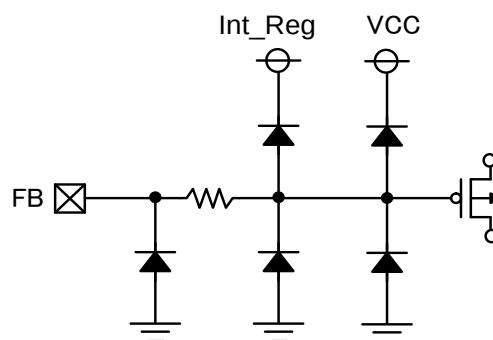
&lt; FB Pin &gt;
