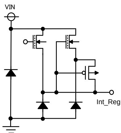
&lt; VIN Pin &gt;
