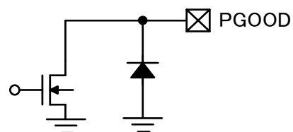
&lt; PGOOD Pin &gt;
