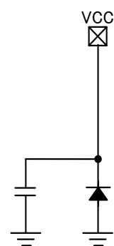
&lt; VCC Pin &gt;
