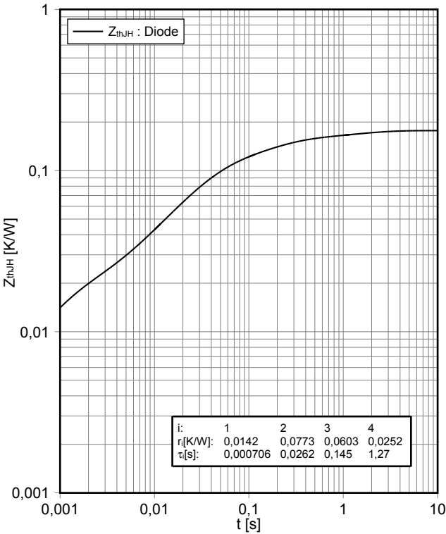
Transienter Wärmewiderstand Diode, Wechselrichter transient thermal impedance Diode, Inverter Z_{thJH} = f(t)
