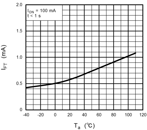
Fig. 12.6 I_{FT} - T_a
