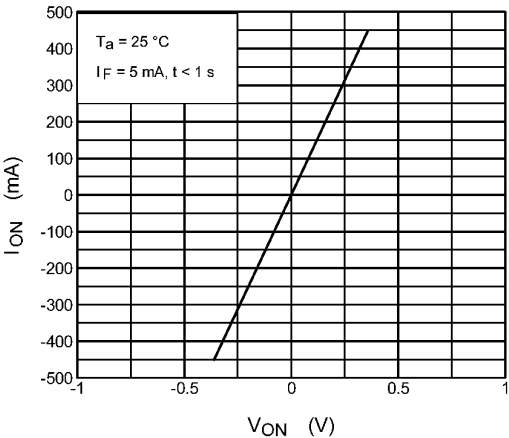
Fig. 12.4 I_{ON} - V_{ON}
