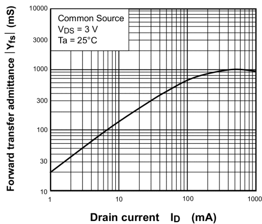
Fig. 7.7 |Y_{fs}| - I_D
