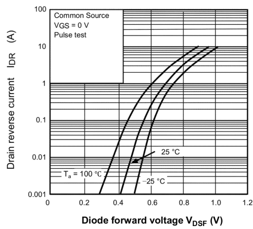
Fig. 8.12 I_{DR} - V_{DSF}
