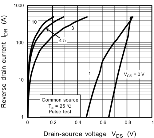
Fig. 8.6 I_{DR} - V_{DS}
