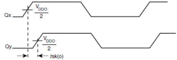
OUTPUT SKEW
