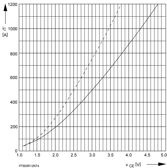
Bild/Fig. 1 Kollektor-Emitter-Spannung im Sättigungsbereich (typisch) Collector-emitter-voltage in saturation region (typical) V_{GE} = 15\text{ V} ----- T_{vj} = 25\text{ °C} —— T_{vj} = 125\text{ °C}
