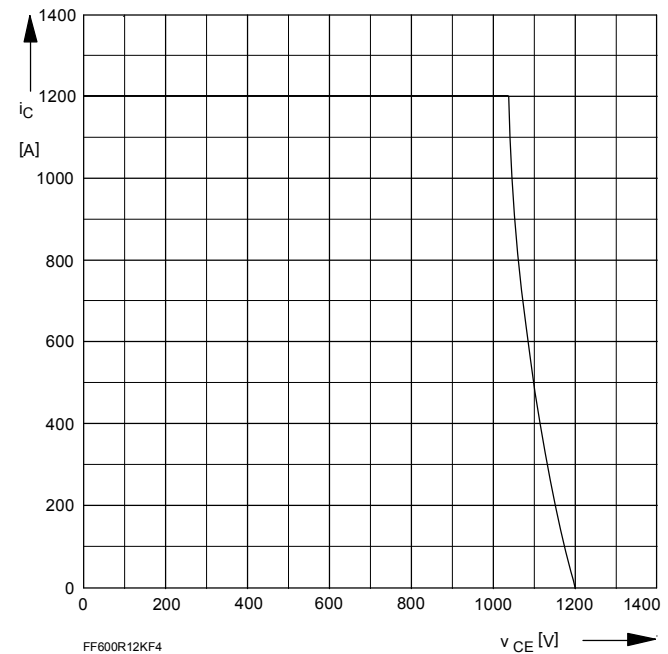
Bild/Fig. 4 Rückwärts-Arbeitsbereich Reverse biased safe operating area t_{vj} = 125\text{ °C} , v_{LE} = v_{LR} = 15\text{ V} , R_G = 1,6\text{ W}
