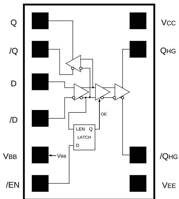
SY10/100EL16VDXC DIE
