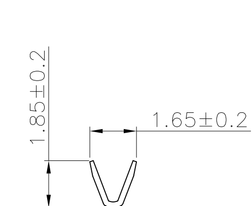
A-A SCALE 2:1
