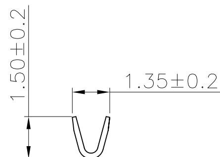
B-B SCALE 2:1
