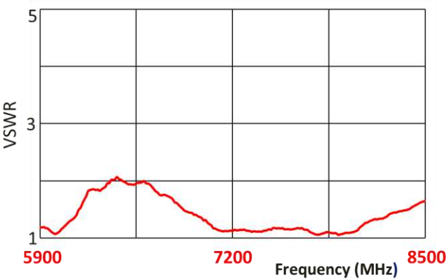
VSWR
