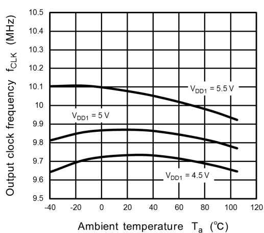
Fig. 12.8 f_{CLK} - T_a
