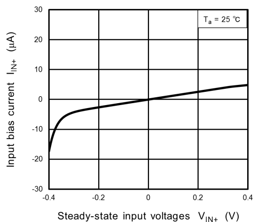
Fig. 12.3 I_{IN+} - V_{IN+}
