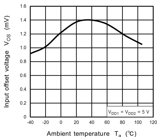
Fig. 12.1 V_{OS} - T_a
