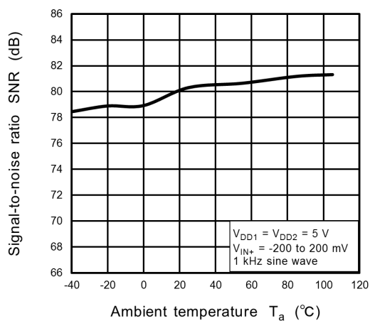
Fig. 12.4 SNR - T_a
