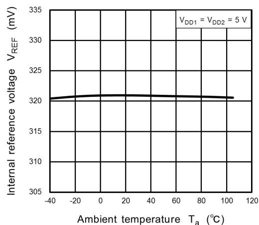
Fig. 12.2 V_{REF} - T_a
