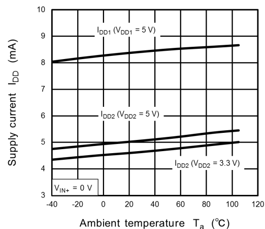
Fig. 12.7 I_{DD} - T_a
