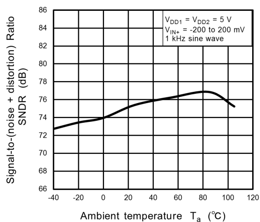
Fig. 12.5 SNDR - T_a
