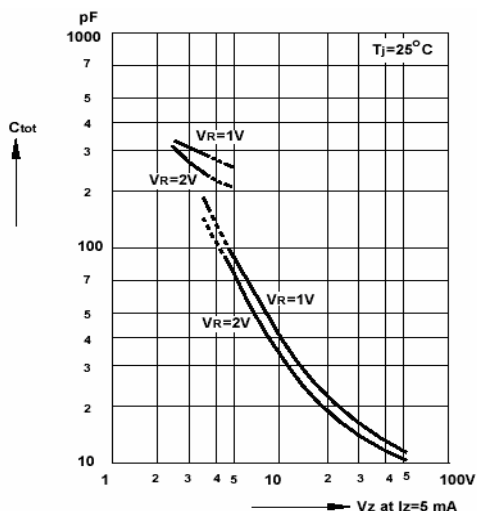
Fig 7. Capacitance vs Zener Voltage
