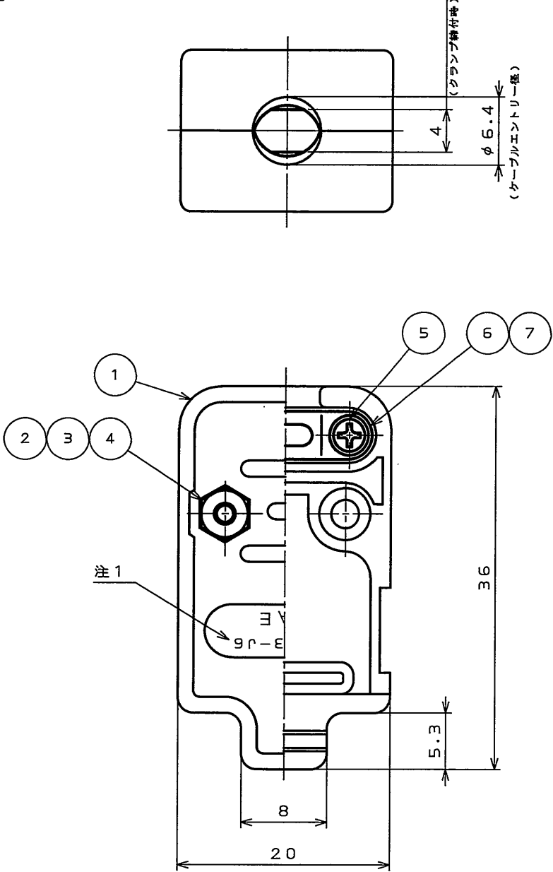
断面 A-A
