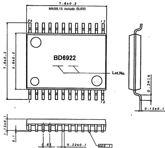
SSOP-B24 (UNIT:mm)
