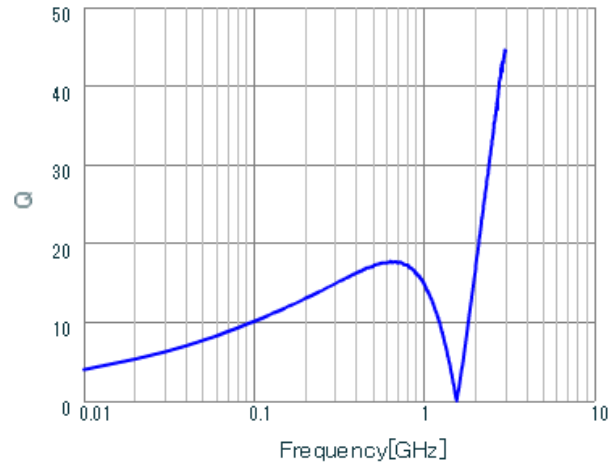
LQG15HN47NH02 Q.
