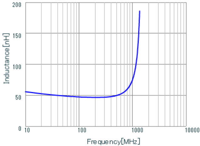
LQG15HN47NH02 L.
