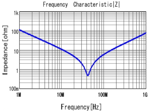
■ DE2E3SA152MA3BT02F |Z| DCOV, 20degC
