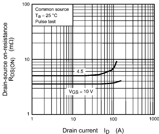
Fig. 8.5 R_{DS(ON)} - I_D
